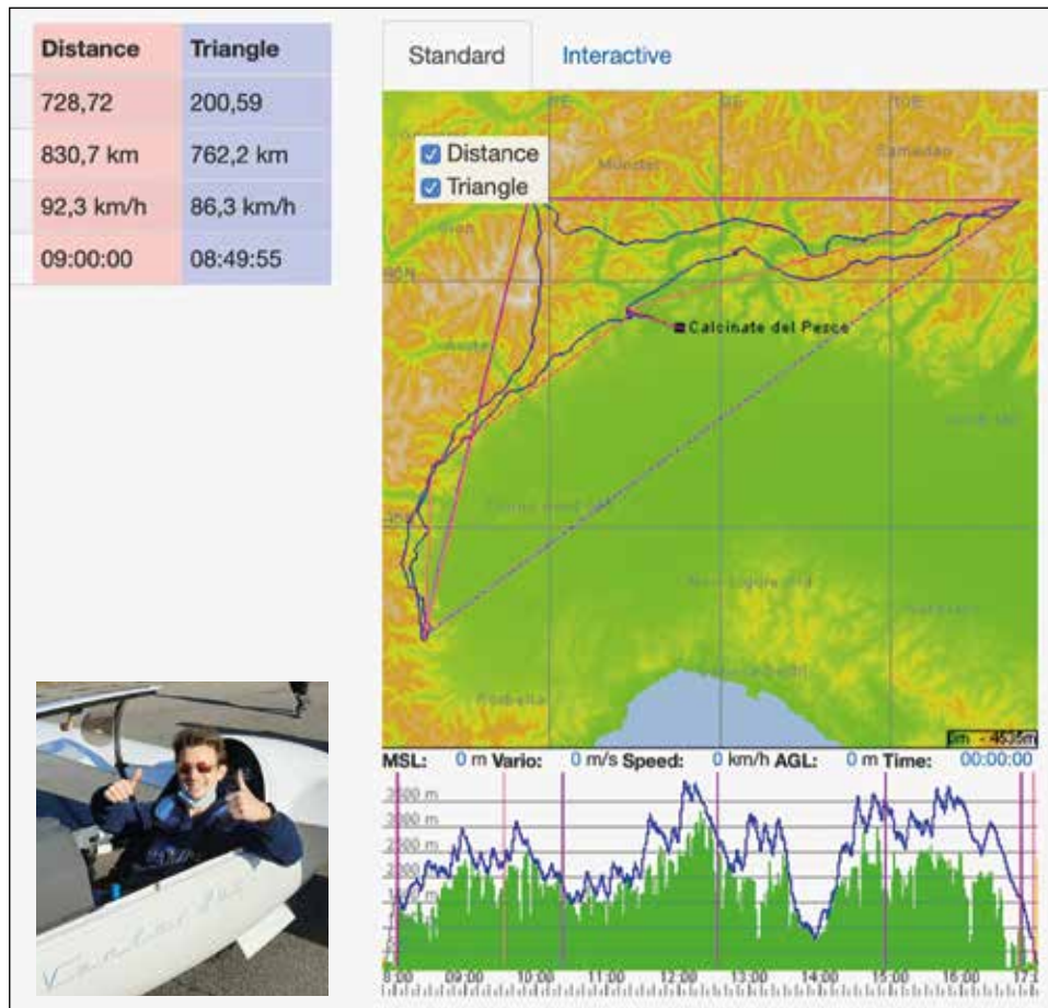
Lorenzo Fornari su Ventus 2 AX Classe 15 m Emilio Bonzanini su Duodiscus Volo da Calcinate di 830,7 km - Triangolo FAI Dichiarato da 762,2 km
